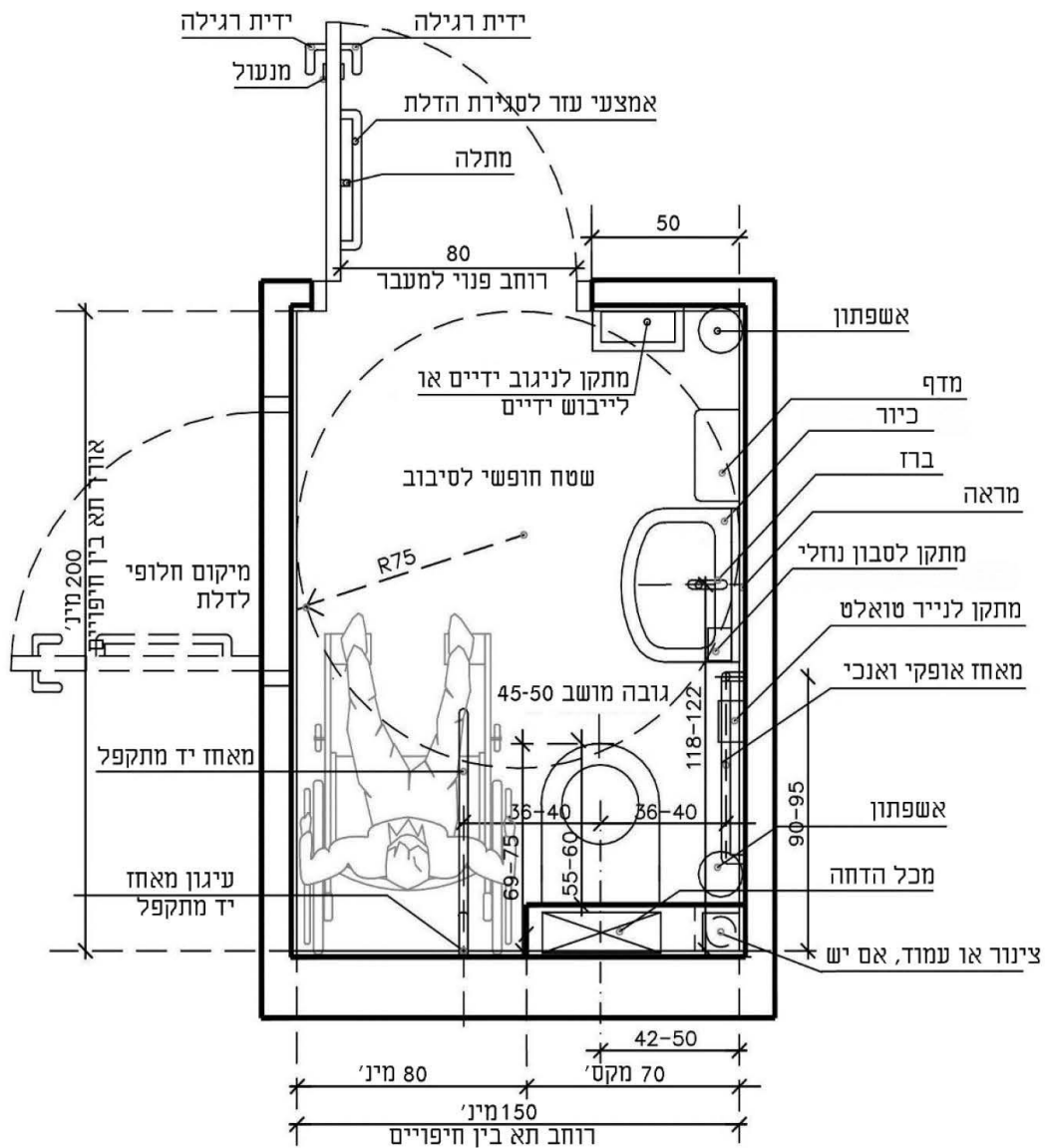
ציור 19 – דוגמות לתאי בית שימוש מטיפוס 1 (המידות בסנטימטרים)
